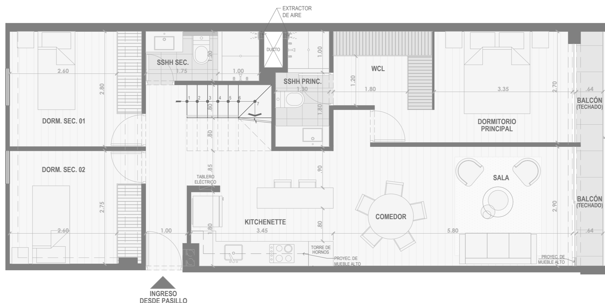
PRIMERA PLANTA (PISO 6)
