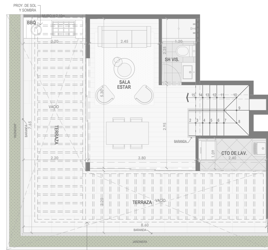
SEGUNDA PLANTA (PISO 7)
